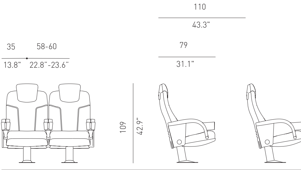
Mod. Mega 9113
