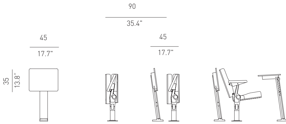
Mod.5072 Minispace+ F48
