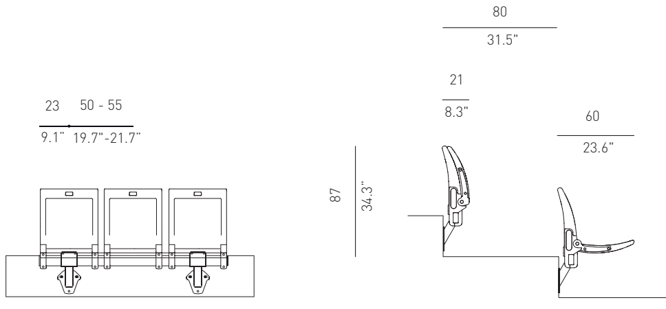
Mod. Arena 303
